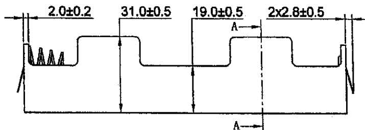
BIG SOLDER LUG S=1.5
