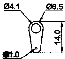
BIG SOLDER LUG S=1.5
