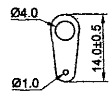
SOLDER LUG S-2
