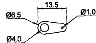
SOLDER LUG S=1:1
