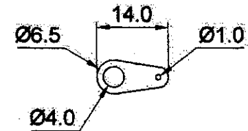
SOLDER LUG
