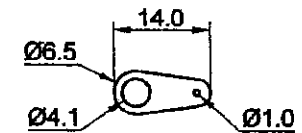
SOLDER LUG S-1
