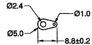
SOLDER LUG
