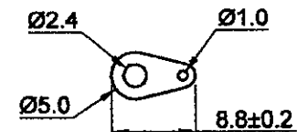
SOLDER LUG
