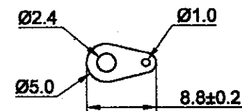
SOLDER LUG
