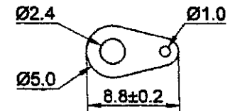
SOLDER LUG
