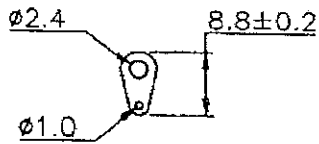
SOLDER LUG
