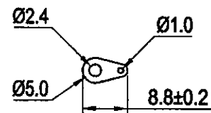
SOLDER LUG
