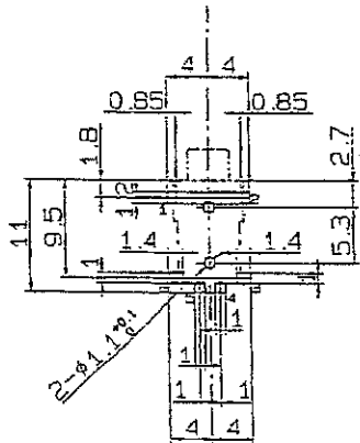
プリント基板半田付け部参考図 (公差±0.1mm) FOOT PRINT
