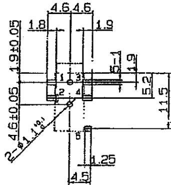
プリント基板半田付け部参照図 FOOT PRINT
