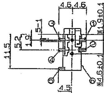
※印は位置決めピンの寸法を示す。
