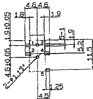
プリント基板半田付け部を示す FOOT PRINT
