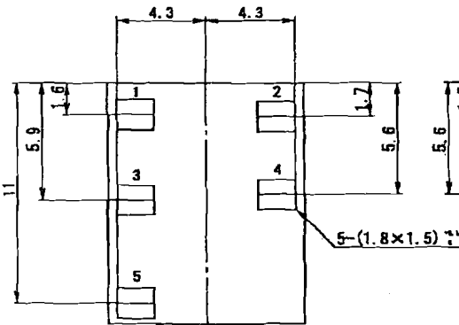
推奨ランド参考図(公差±0.1mm, 実装面側より見る) Reference drawing of recommendation land (Tolerance ±0.1mm : Seen from mounting side.)
