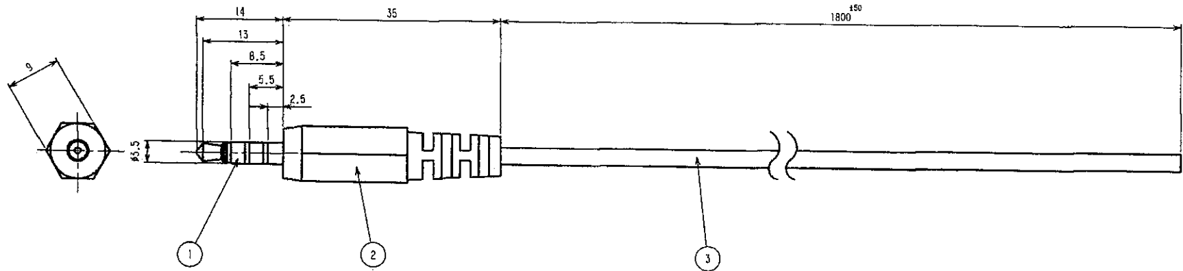
ケーブル仕様
