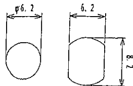
取付穴参考寸法
