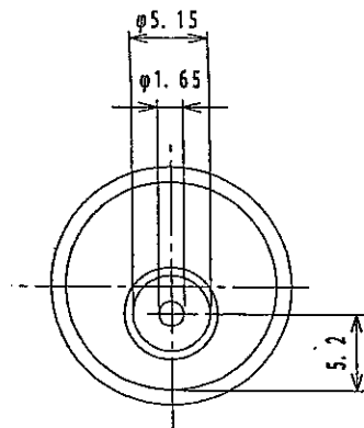
取付穴参考寸法
