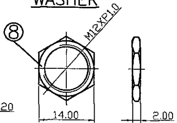
NUT
