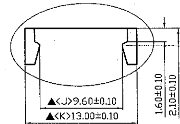
A部詳圖: (塑柱 2/1)
