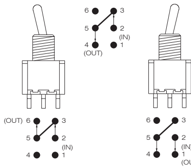
SP3T
