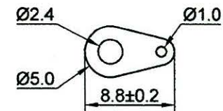
SOLDER LUG
