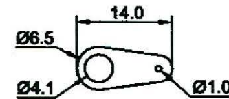
BIG SOLDER LUG S=2
