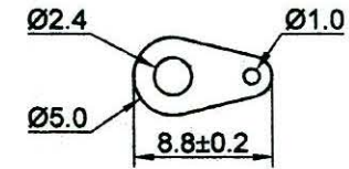
SOLDER LUG
