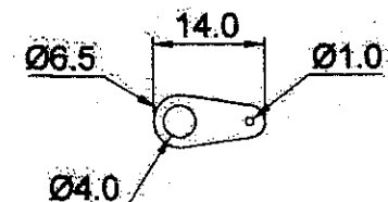
SOLDER LUG
