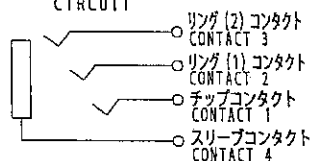
回路図
