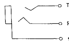
回路図
