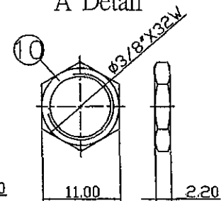
NUT
