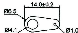
SOLDER LUG S=3
